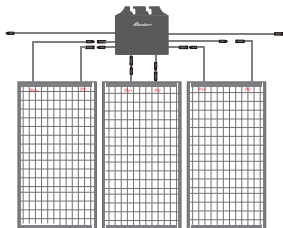
AW-PVRS-A3/B3/C3 1:3 连接示意图
