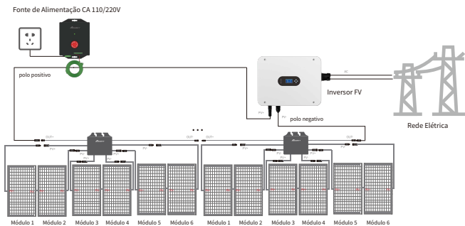
AW-PVRS-A6/B6/C6 1:6 Diagrama de Conexão do Controlador
