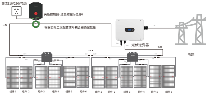
AW-PVRS-A6/B6/C6 1.6 控制器连接示意图
