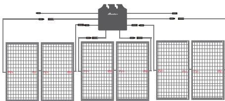
AW-PVRS-A6/B6/C6 1:6 Diagrama de Conexão de Cadeias Fotovoltaicas em Paralelo
