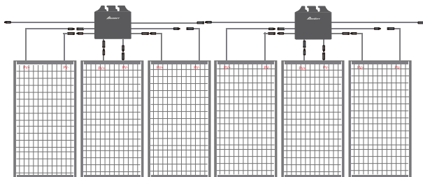
AW-PVRS-A3/B3/C3 1:3 Diagrama de Conexão do Controlador
