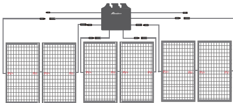
AW-PVRS-A6/B6/C6 1:6 连接示意图
