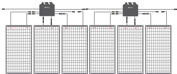
AW-PVRS-A3/B3/C3 1:3 组串并联连接示意图
