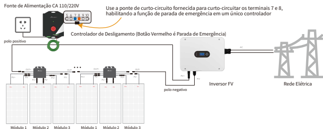
AW-PVRS-A3/B3/C3 1:3 Diagrama de Conexão do Controlador
