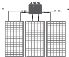
AW-PVRS-A3/B3/C3 Diagrama de Conexão 1:3
