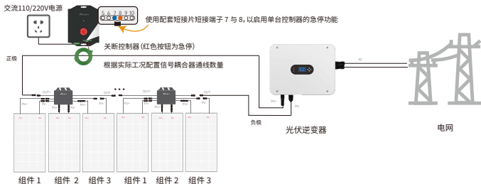
AW-PVRS-A3/B3/C3 1:3 控制器连接示意图
